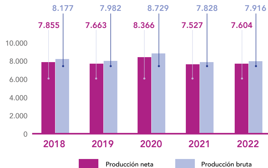
CN. ALMARAZ UII - Producción (GWh)
