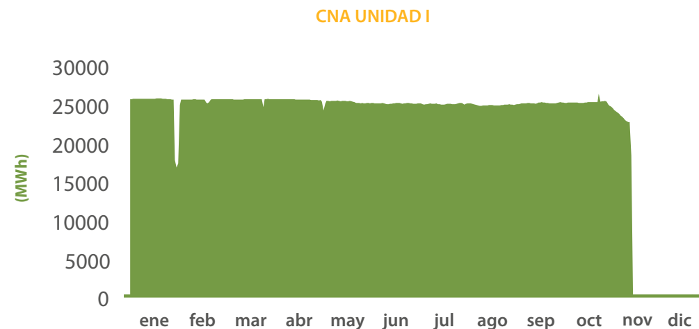
CN ALMARAZ PRODUCCIÓN DIARIA 2021
