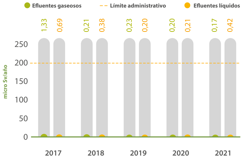
DOSIS EFECTIVA AL EXTERIOR POR EFLUENTES CN. ALMARAZ
